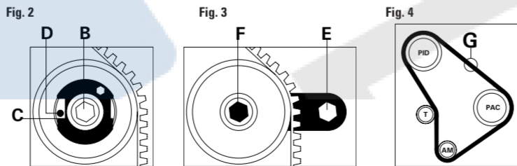
FIGURA 2 Per motori non turbo: allentare il bullone di bloccaggio B e ruotare in senso orario il tendicinghia fino ad allineare la tacca C con la tacca D, quindi, serrare il bullone di bloccaggio B.
