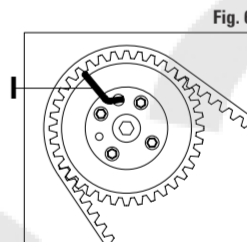
FIGURA 6 Inserire l'apposito attrezzo di bloccaggio I, della puleggia della pompa di iniezione.
