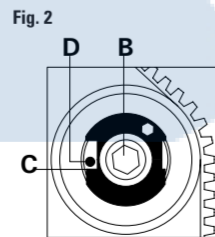
FIGURA 2 PARA MOTORES TURBO: Aflojar el tornillo de fijación B y luego girar el tensor de correa en sentido de las agujas del reloj hasta lograr alinear la marca C con la marca D. Por último, apretar el tornillo de fijación B.
