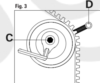
FIGURA 3 Aflojar el tornillo de fijación C. Suelte el tensor de correa hasta la obtención de la tensión correcta. Apretar el tornillo de fijación C. Asegurarse que el resorte D quede insertado con su respectivo tornillo de fijación.
