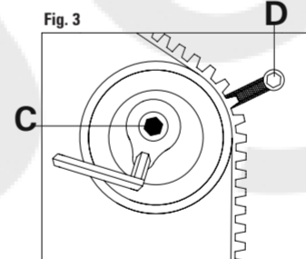
FIGURA 3 Allentare il bullone di bloccaggio C e rilasciare il tendicinghia fino alla corretta tensione, quindi serrare il bullone di bloccaggio C. Assicurarsi che sia inserita la molla D con l'apposito pino di fissaggio.
