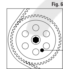
FIGURA 6 Insertar la herramienta para inmovilización de polea de bomba de inyección H.
