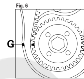
FIGURA 6 Controllare il corretto allineamento delle tacche di fase G. FIGURA 7 Inserire l'apposito attrezzo di bloccaggio del volante H.
