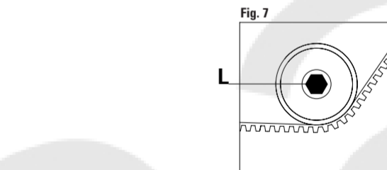
FIGURA 7 Allentare il bullone di bloccaggio del tendicinghia della pompa di iniezione L e lasciare agire il tendicinghia fino alla giusta tensione; serrare, quindi, il bullone di bloccaggio L.
