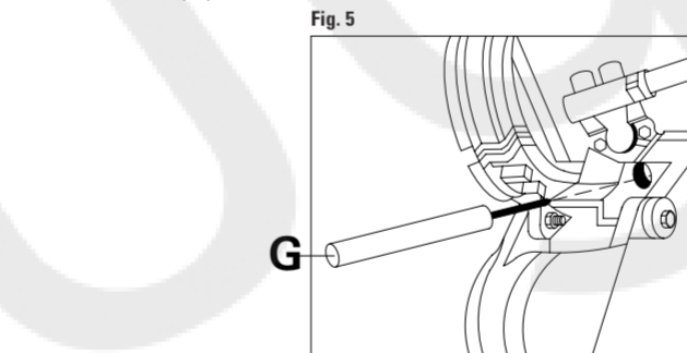
FIGURA 5 Insertar la herramienta inmovilizadora de cigüeñales G, y asegurarse de que el brazo del cigüeñal apoye sobre la herramienta.
