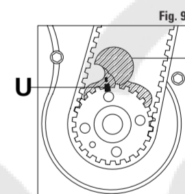
FIGURA 9 La tacca di fasatura sull'attrezzo di bloccaggio T, deve essere allineata con la tacca di fasatura dell'albero motore U.
