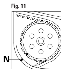
FIGURA 10 Verificar la correcta alineación de las marcas de fase M (Bomba Bosch). FIGURA 11 Verificar la correcta alineación de las marcas de fase N (Bomba Lucas). FIGURA 12 Insertar la herramienta de inmovilización de la bomba de inyección O.
