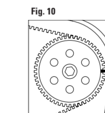
FIGURA 10 Controllare il corretto allineamento delle tacche di fase M (pompa Bosch). FIGURA 11 Controllare il corretto allineamento delle tacche di fase N (pompa Lucas). FIGURA 12 Inserire l'apposito attrezzo di bloccaggio della pompa di iniezione O.
