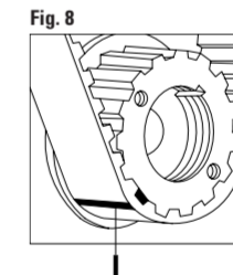
FIGURA 8 Controllare il corretto allineamento delle tacche di fase I. FIGURA 9 Inserire l'apposito attrezzo di bloccaggio dell'albero motore L.
