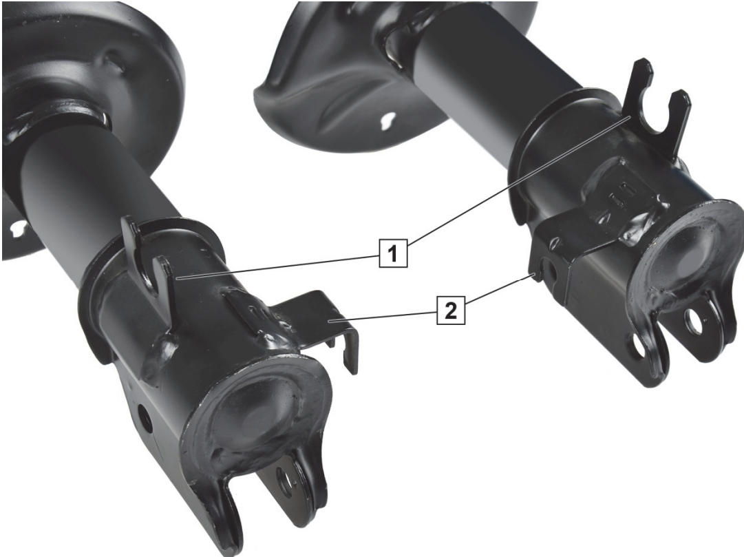
Abb./Fig. 1: Stoßdämpfer mit Haltern / Shock Absorber with brackets / Amortisseur avec fixations / Amortiguador con soportes
