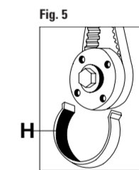
FIGURA 4 Insertar la herramienta de inmovilización del volante motor G. FIGURA 5 Insertar la herramienta específica para inmovilizar la correa de distribución H. FIGURA 6 Verificar la correcta alineación de las marcas de puesta en fase I.
