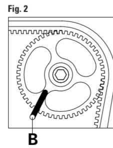
FIGURA 1 Insertar la herramienta especial de inmovilización de árbol de levas A. FIGURA 2 Insertar la herramienta especial de inmovilización de árbol de levas B.
