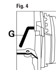
FIGURA 4 Inserire l'apposito attrezzo di bloccaggio del volante G. FIGURA 5 Inserire l'apposito attrezzo di bloccaggio della cinghia di distribuzione H. FIGURA 6 Controllare il corretto allineamento delle tacche di fase I.
