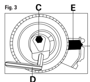
FIGURA 3 Allentare il bullone di bloccaggio, C, e ruotare il tendicinghia in senso antiorario tramite la chiave esagonale D, quindi, allineare l'indicatore, E, al centro della zona di controllo, F, serrare quindi il bullone di bloccaggio C.
