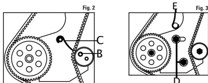
FIGURA 2: Allentare il bullone di bloccaggio B, inserire la molla C del tendicinghia, togliere gli attrezzi di bloccaggio e far ruotare l'albero motore in senso antiorario di 60°; serrare quindi il bullone di bloccaggio B. FIGURA 3: Allentare i bulloni di bloccaggio D, inserire la molla E del tendicinghia, togliere gli attrezzi di bloccaggio e far ruotare l'albero motore in senso antiorario di 60°; serrare quindi i bulloni di bloccaggio D.
