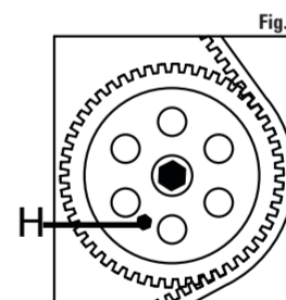
FIGURA 6: Inserire la ferramenta para inmovilización de polea de bomba de inyección H. Tornillo M8 x 1.25.
