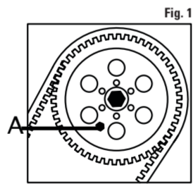
FIGURA 1: Insertar la herramienta inmovilizadora de árbol de levas A. Tornillo M6 x 1.00.
