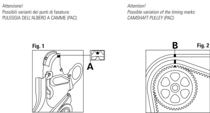
FIGURA 1 Controllare il corretto allineamento della tacca di fasatura, verificando che risulti allineata al carter distribuzione A. FIGURA 2 Controllare il corretto allineamento delle tacche di fase B.
