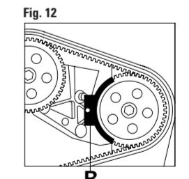
FIGURA 11 Verificar la correcta alineación de las marcas de fase Q. FIGURA 12 Insertar la herramienta para inmovilización de polea de bomba de inyección R.
