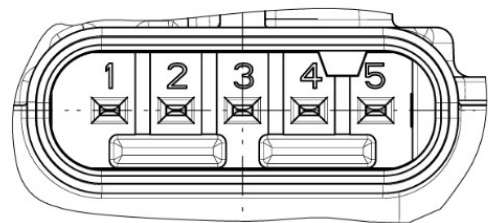
2 - Anschluss / Connector
